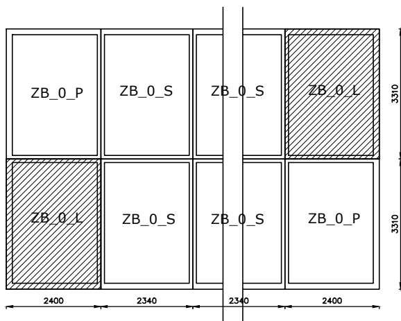
SCHEMAT ZBIORNIKÓW
